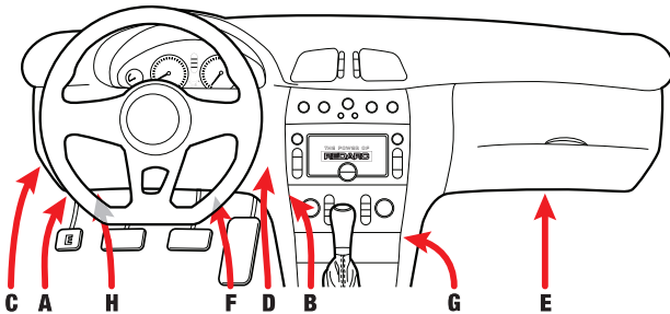
Image A - Common connector locations Image A - Emplacements usuels du connecteur Imagen A - Ubicaciones habituales del conector
