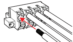
Image C - Tow-Pro Classic Connector (Green) Image C - Connecteur Tow-Pro Classic (vert) Imagen C - Conector de Tow-Pro Classic (Verde)
